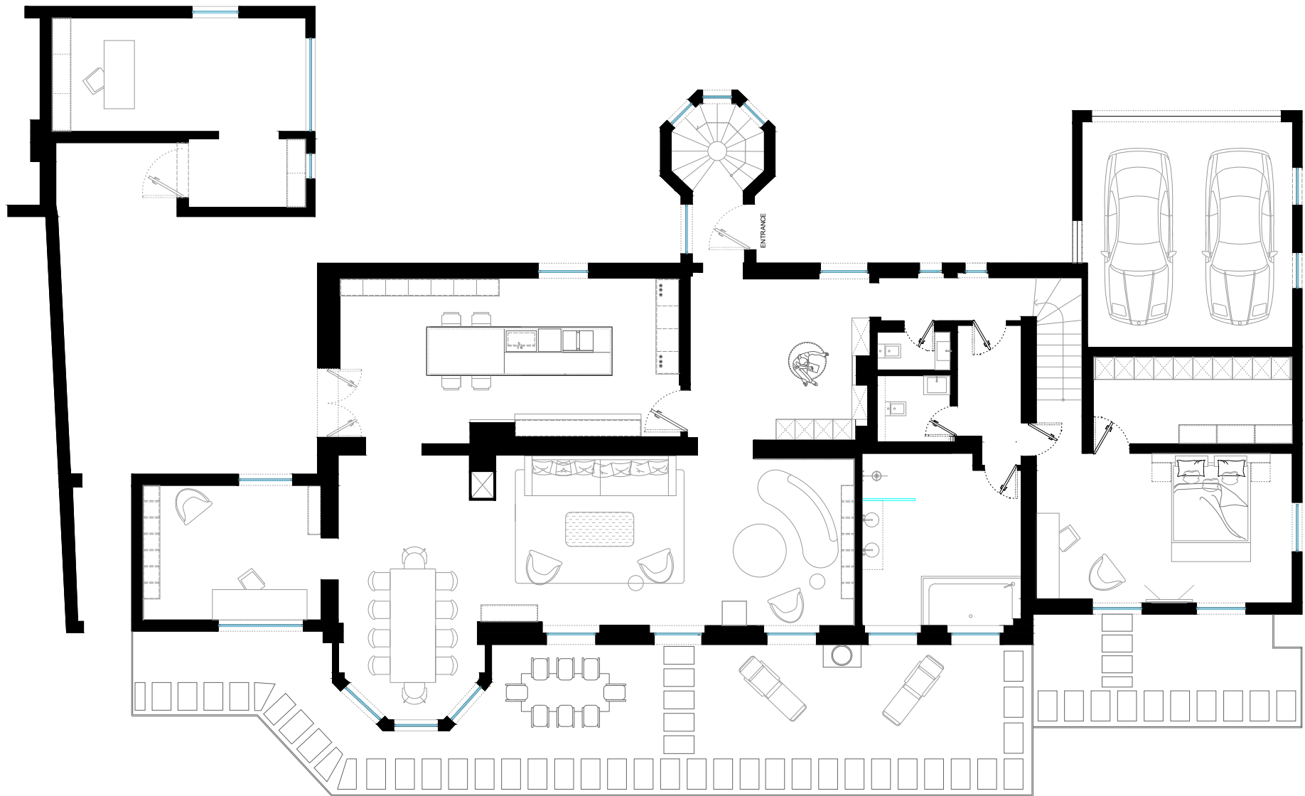
Erdgeschoss
